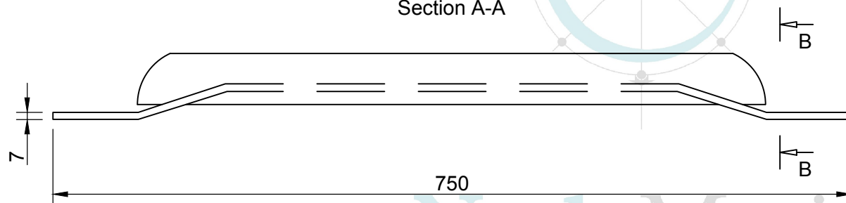
Section A-A
