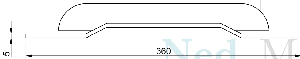
Section A-A
